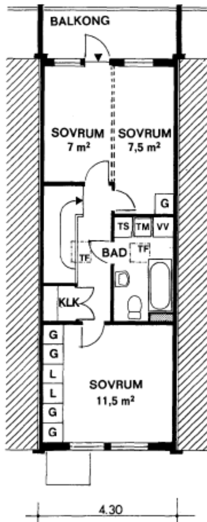
ÖVERPLAN
